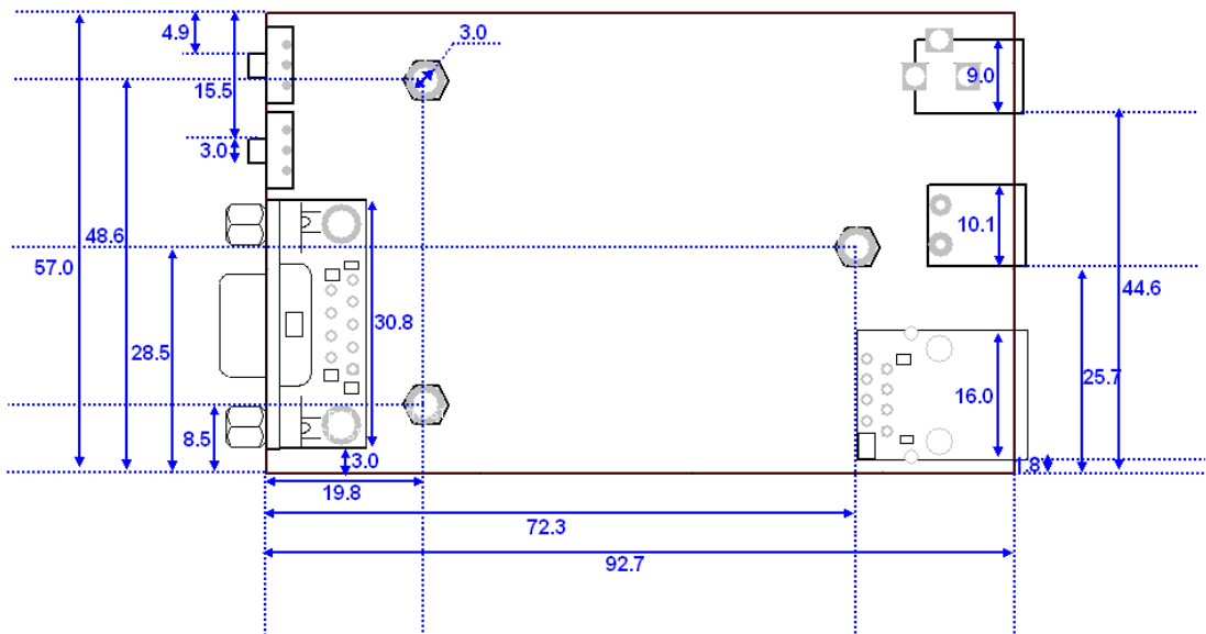
图 4 ZLSN5102 尺寸图
