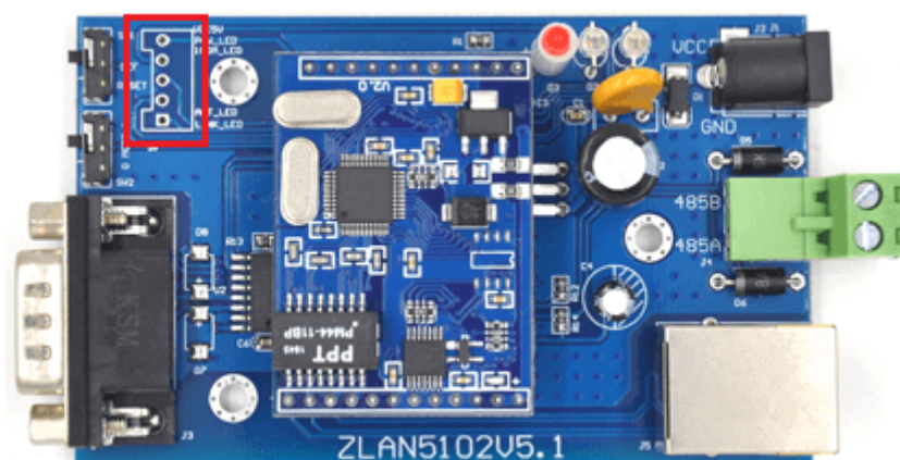
图 1 ZLSN5102 联网模块
